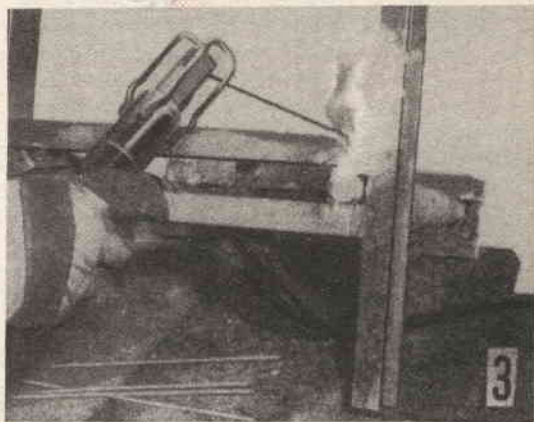
Saldatura lungo le linee di contatto tra i quattro elementi che compongono la base della pressa.
