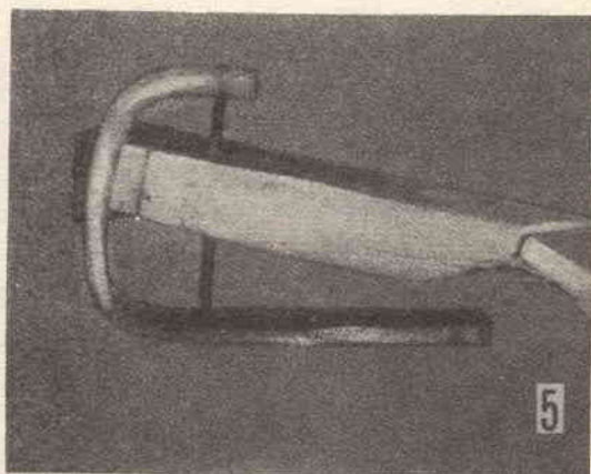
Veduta ravvicinata del supporto per il perno, del perno stesso, e della parte terminale del braccio del pick up; alla estrema destra, lo snodo tra le due sezioni del braccio, realizzato con la striscetta di pelle.
